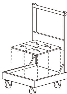
一斗缶台車 LRO-58 ¥163,000 580×580×550(mm) ※特注サイズにも対応いたします。
